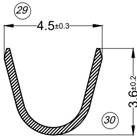
SECC. C-C
